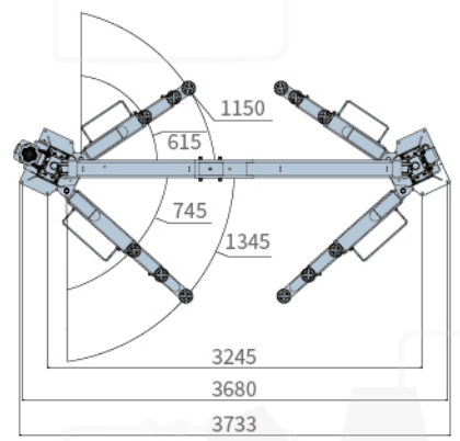
不对称款
