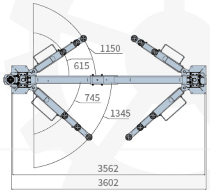
对称款
