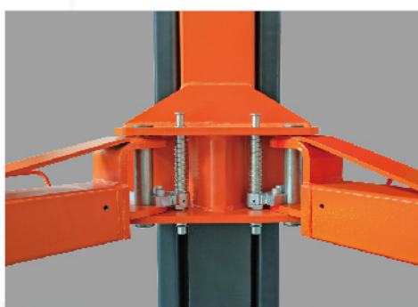
举升臂自锁装置
