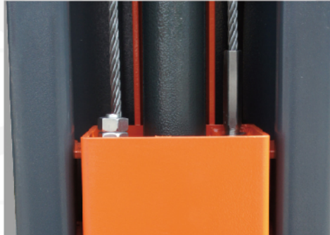
珩磨管油缸，预拉伸钢芯钢丝绳
