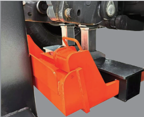
高杆支架和支撑梁（选配）
