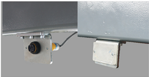
红外同步保护装置，防止车辆侧翻
