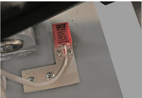
下降防压蜂鸣器 (一次平台离地500mm，自动报警)
