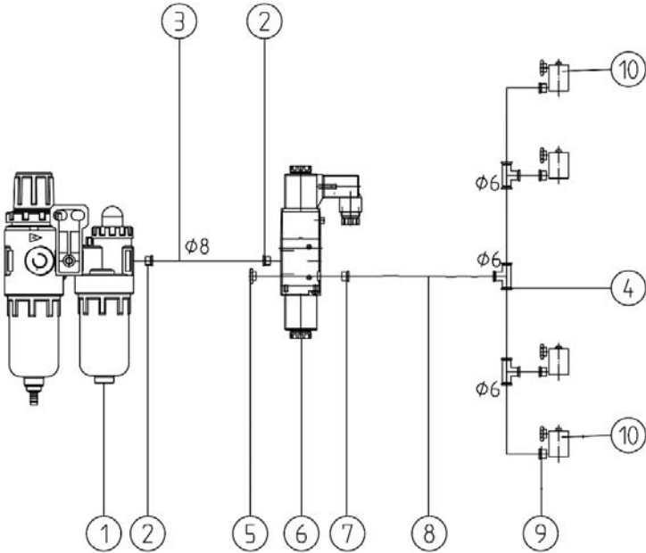
附件 3，氣動原理圖及元件清單
