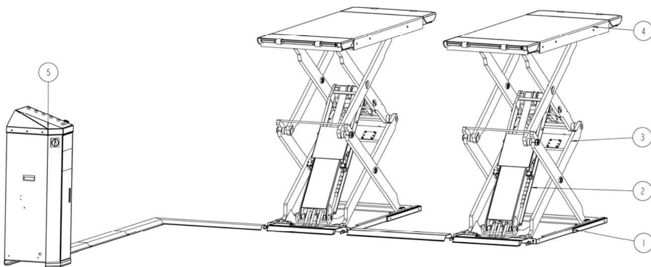
1.底板组件 2.油缸组件 3.支架组件 4.举升平台 5.控制柜
