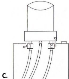
C. 一調平閥打開，一個調平閥關閉：調平狀態
