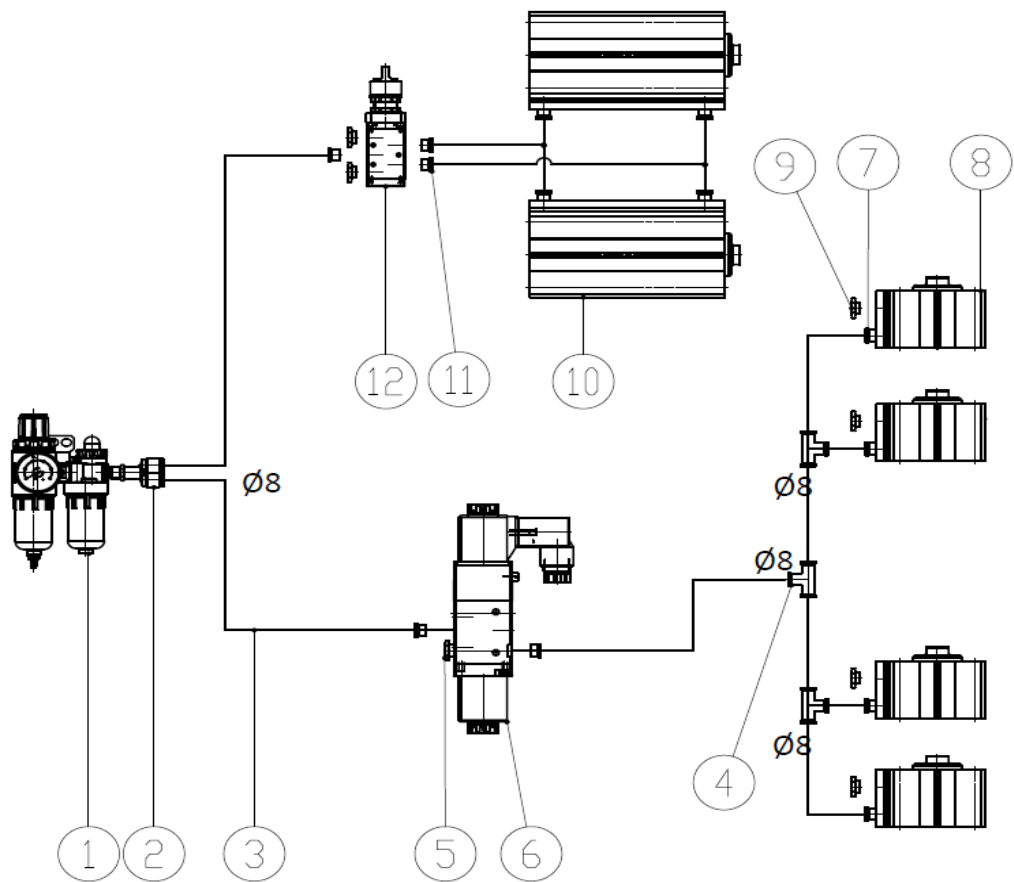
附件 4、气动原理图及元件清单
