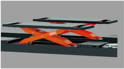
二次举升双抽拉小车 (子剪举升吨位3500kg) BWF款
