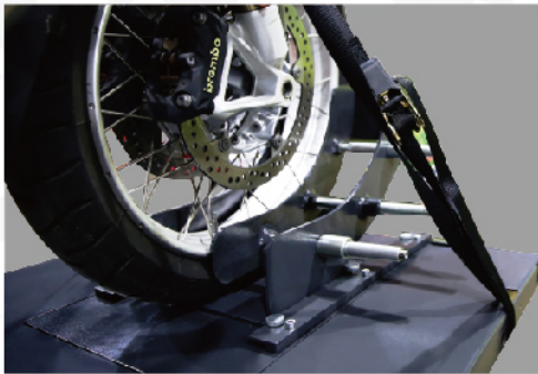
手动夹具
